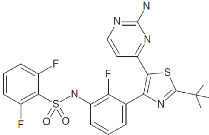
Abbildung 3 Molekulare Struktur des BRAF-Inhibitors Dabrafenib.
